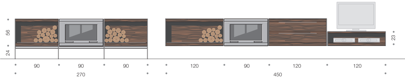
Kombinationsbeispiel: Kaminofen mit Stauraumelementen aus Holz Sample combination: stove with wooden storage element Kombinationsbeispiel: Kaminofen mit Stauraumelement, Schubkastenelement und TV-Konsole aus Holz Sample combination: stove with storage element, drawer element and TV console in wood
