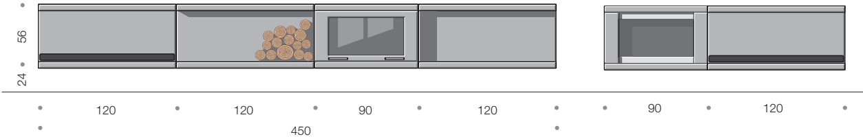
Kombinationsbeispiel: Kaminofen mit Stauraumelementen und Bank Sample combination: stove with storage elements and bench Kombinationsbeispiel: Alkohol-Kamin mit Bank Sample combination: alcohol-fuelled fireplace with bench
